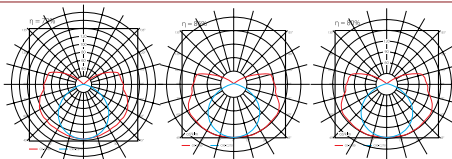
Világítási diagram / Lighting curve
