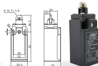
ST11032 - Görgős végálláskapcsoló / Roller plunger type
