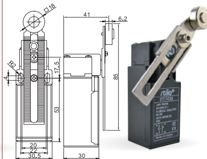
ST11035 - Állítható karos-görgős végálláskapcsoló / Adjustable roller arm type
