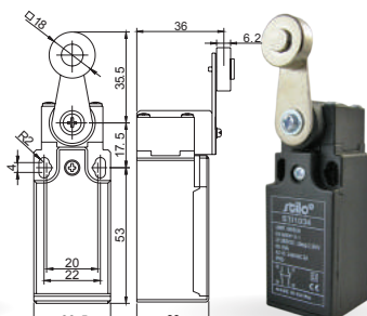
ST11034 - Karos-görgős végálláskapcsoló / Roller arm type
