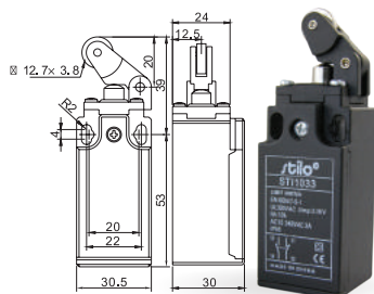
ST11033 - Egyirányú működtetésű görgős végálláskapcsoló / Roller lever type
