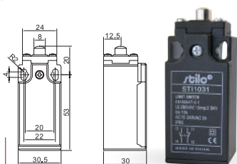
ST11031 - Büttykös végálláskapcsoló / Push plunger type
