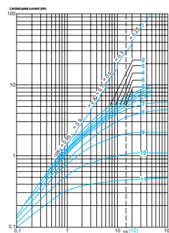
Áramkorlátozási jelleggörbe / Current limit characteristic
