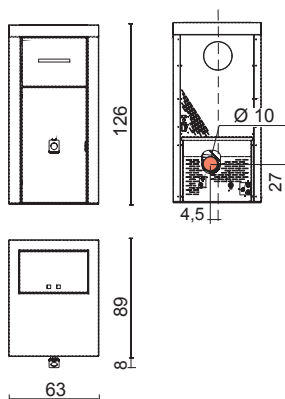
FATÜZELÉSŰ KAZÁN Energy Plus 21/26/30/34
