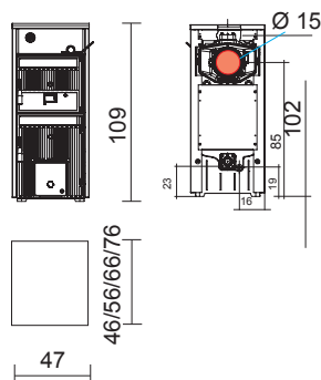
FATÜZELÉSŰ KAZÁN Energy Plus 21/26/30/34
