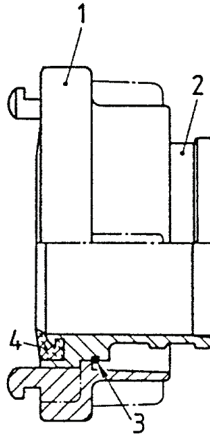
Tömlőkapocs kialakítása
